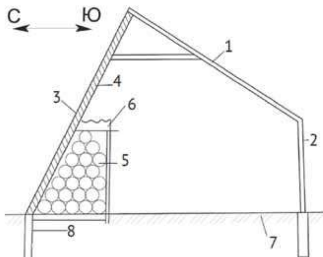
Рис.: 1 - прозрачная изоляция, 2 - опорная стенка, 3 - северная стена, 4 - теплоизоляция, 5 - галечный аккумулятор, 6 - ящики с рассадой, 7 - защищенный грунт, 8 - теплоизолированный фундамент.
