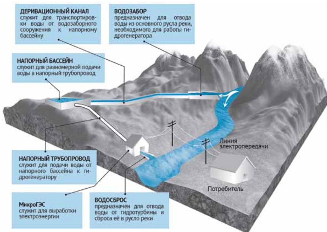
Рис. 3.1.12. Принцип действия малой ГЭС
