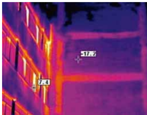
Рис. 3.2.14. Фотография в инфракрасных лучах показывает, насколько эффективнее теплоизоляция пассивного дома (справа) по сравнению с обычным домом (слева). Фото потерь тепла в здании школы. (фото сделано в рамках работ проекта SPARE Кыргызстане)
