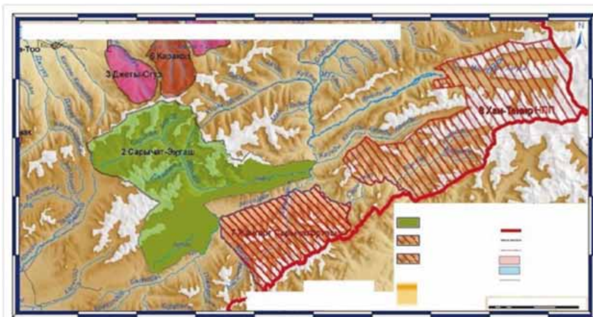
Рис. 2.2.3. Карта ООПТ Иссык-Кульской области.
