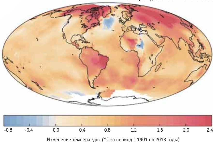
Рис. 1.1. Карта наблюдаемых изменений приземной температуры с 1901 по 2013 годы.
