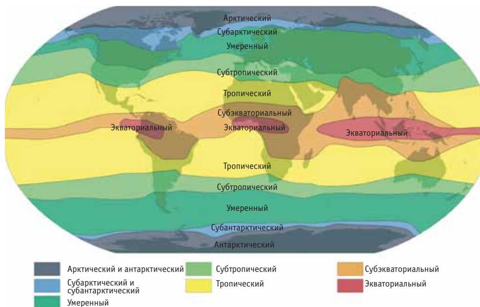
Рис. 1.2.2. Карта климатических поясов Земли по Б. П. Алисову.
