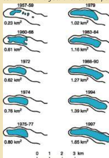
Рис. 2.7.19. За последние 50 лет оз. Тшо Ролпа увеличилось в 7 раз.
