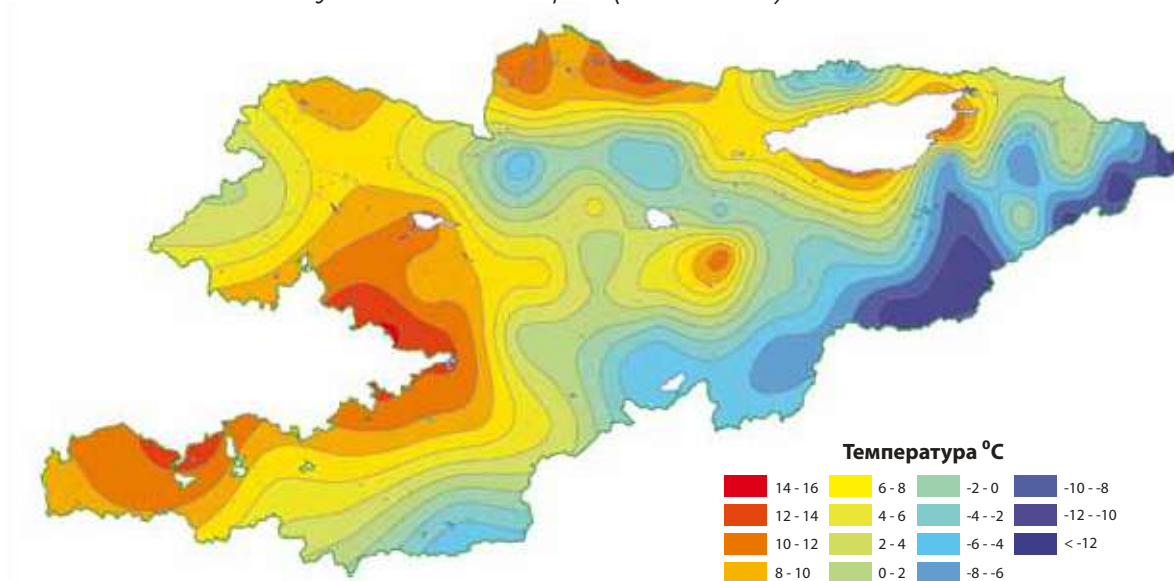
Рис. 1.4.8. Распределение среднегодовой температуры на территории Кыргызской Республики за базовый период (1961-1990 гг.).
