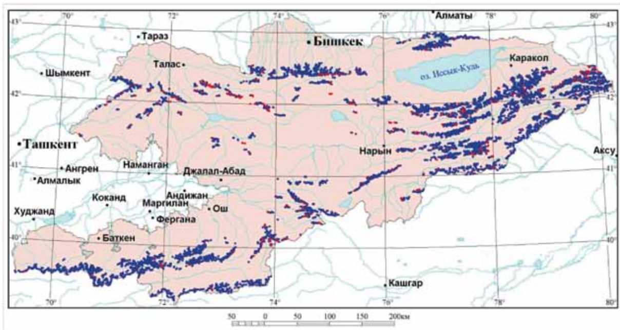
Рис. 2.4.4. Изменение площади оледенения к 2000 году относительно 1960-х годов.
