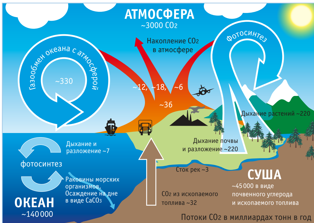
Рис. 1.4.5. Круговорот \text{CO}_2 в природе.
