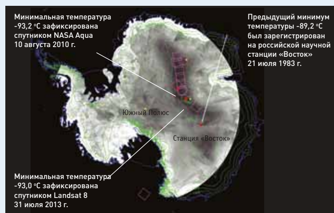
Рис. 1.2.7. Данные о температуре воздуха у поверхности Антарктиды, полученные с американских спутников NASA Aqua в 2003–2013 годах и Landsat 8 в 2013 году.
