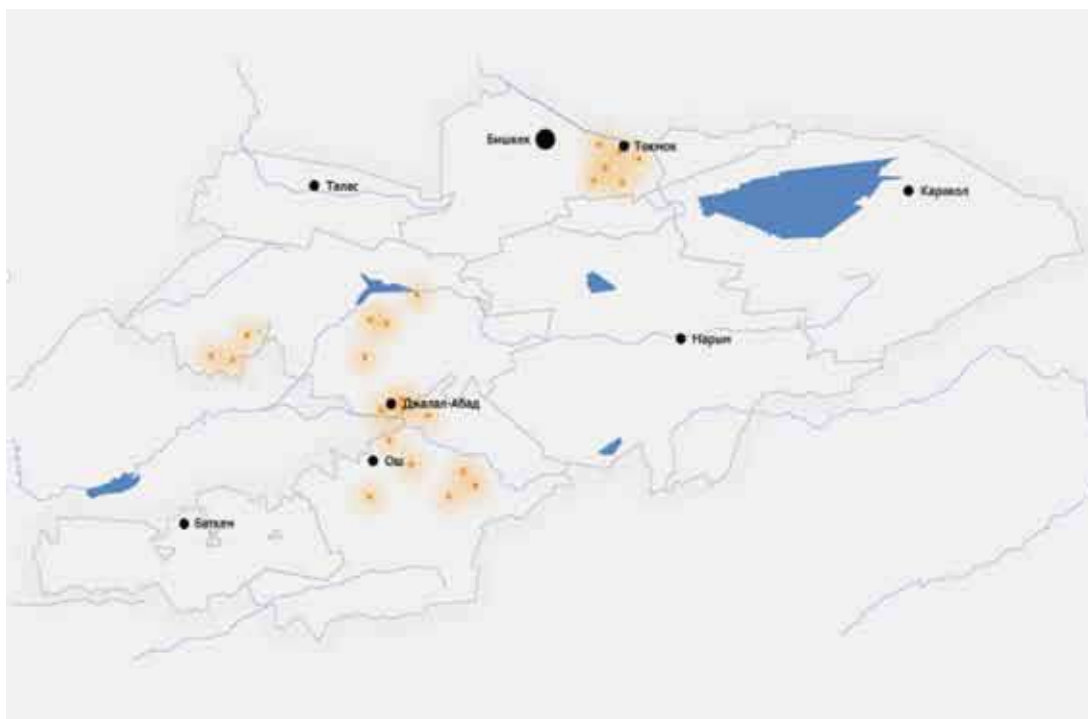
Рис. 2.7.17. Пострадавшие от селя регионы Кыргызстана и материальный ущерб.
