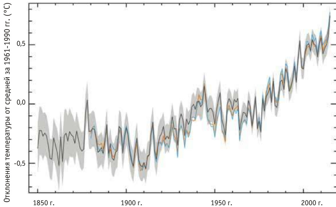
Рис. 1.4.6. Рост средней температуры воздуха на Земле с 1850 по 2015 годы.
