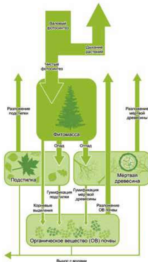
Рис. 2.3.11. Схема бюджета углерода
