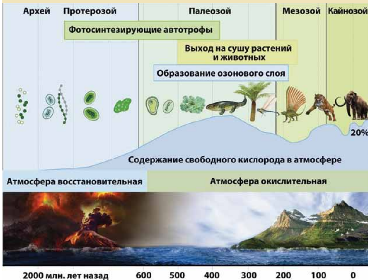
Рис. 2.2.1. Смена типов атмосфер и появление возможности выхода на сушу высших растений и животных
