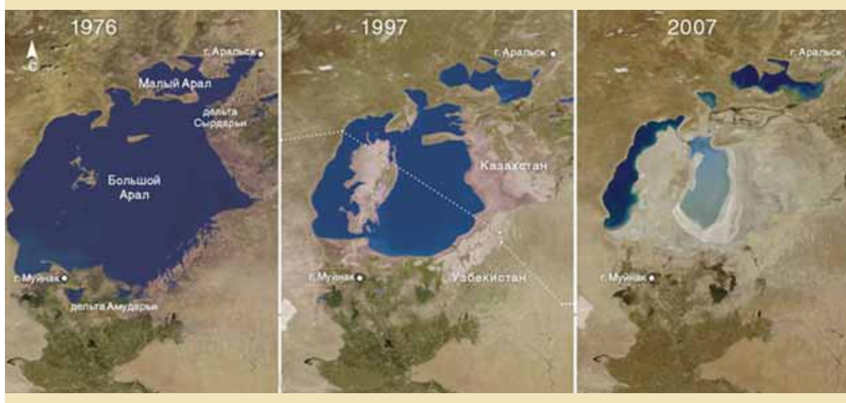
Рис. 2.4.9. Аральское море в Центральной Азии.
