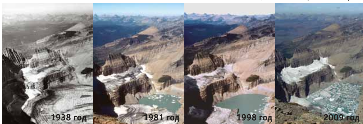
Рис. 2.7.13. Таяние ледника Гриннел в Национальном парке «Глейшер».
