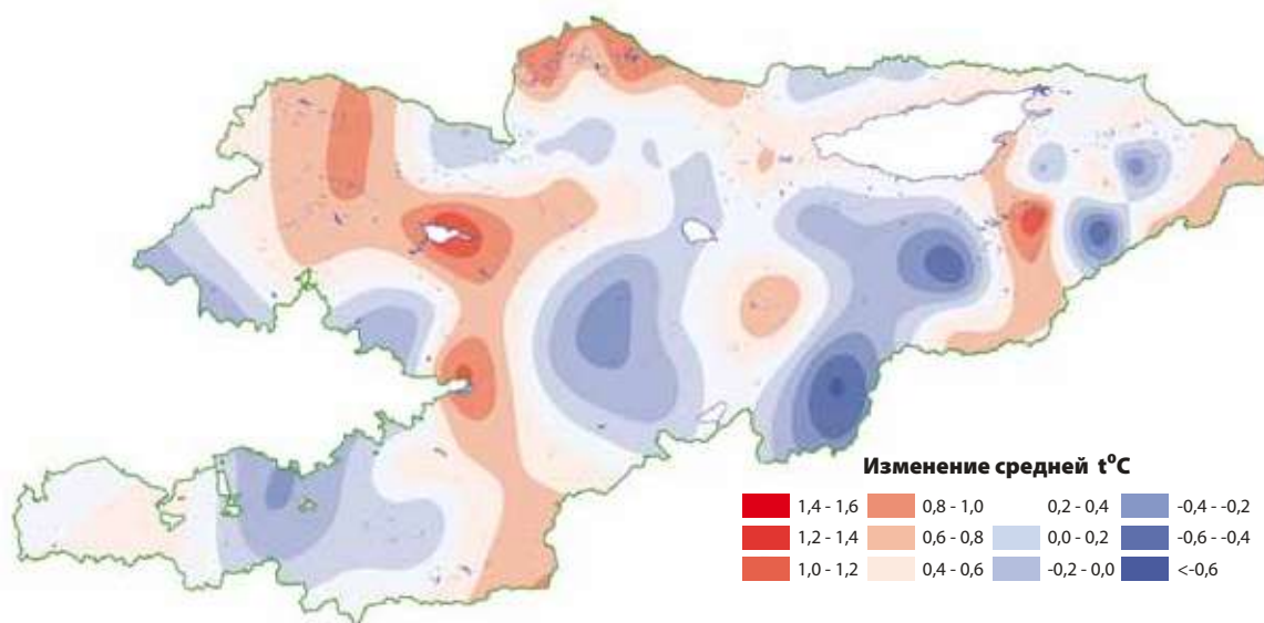
Рис. 1.4.9. Распределение зон различной скорости роста среднегодовой температуры в °С за последние 20 лет по отношению к периоду (1961-1990 гг.).
