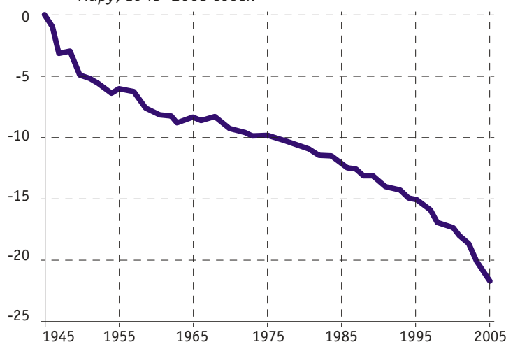
Рис. 2.7.5. Изменение массы горных ледников по всему миру, 1945–2005 годы.
