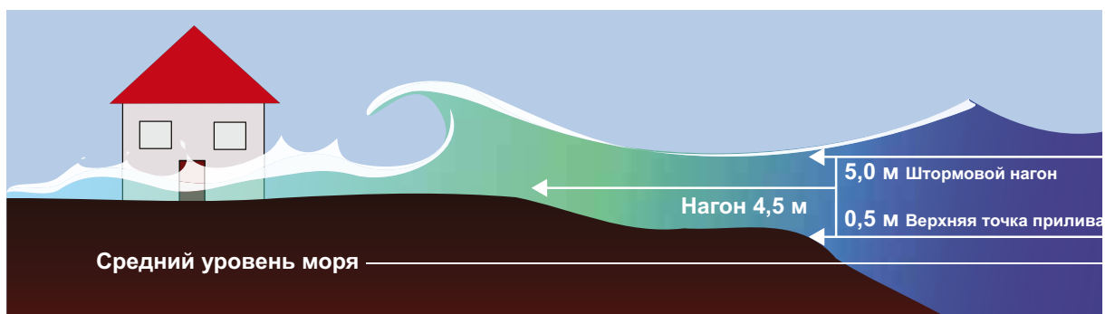
Рис. 2.6.2. Штормовой нагон.
