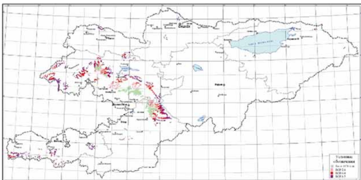
Рис. 2.3.6. Ареалы для арчи зеравшанской
