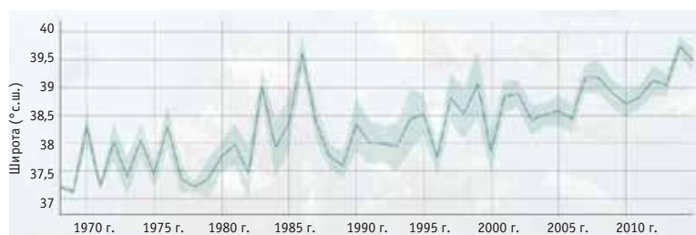
Рис. 2.6.8. Чёрный морской окунь смещается на север по мере роста температуры океана.
