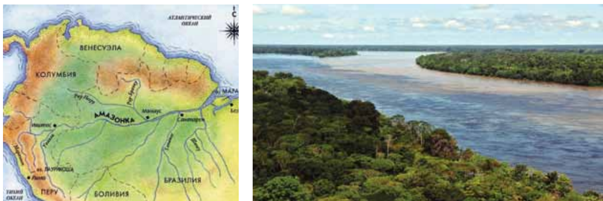
Рис. 2.4.7. Самый большой водосборный бассейн у р. Амазонки в Южной Америке – его площадь составляет 7 млн км 2 .
