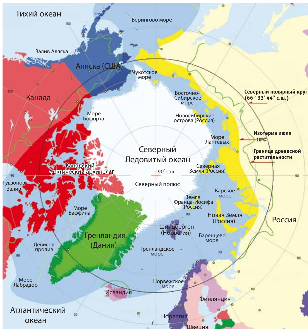
Рис. 2.8.1. Определение границ Арктики.
