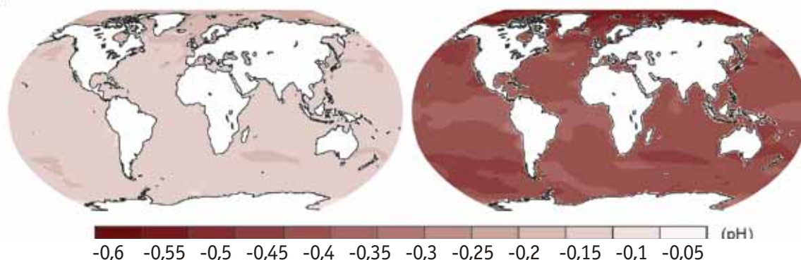
Рис. 2.6.7. Прогноз изменения кислотности поверхности океана к концу XXI века при наиболее благоприятном (слева) и наименее благоприятном (справа) сценариях воздействия человека на климатическую систему.
