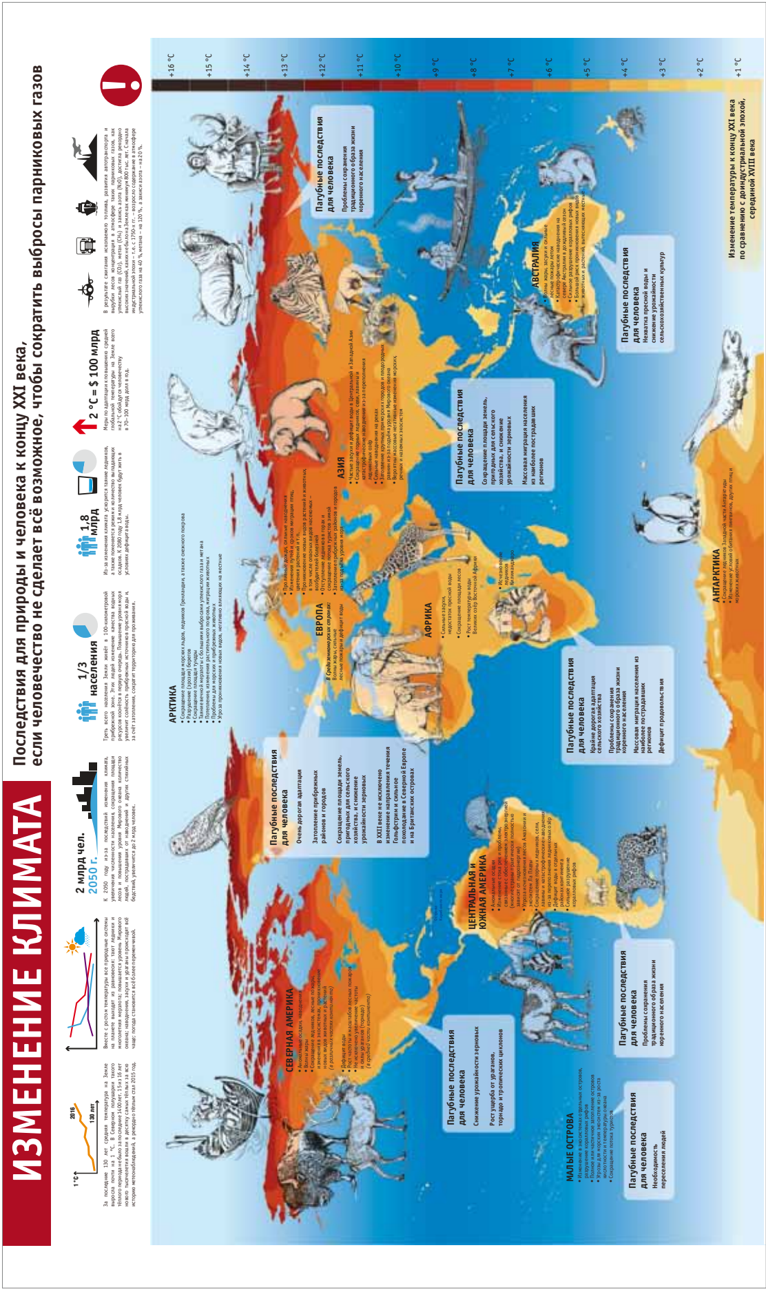
Рис. 2.1. Изменения климата: последствия для природы и человека к концу XXI века, если человечество не сделает всё возможное, чтобы сократить выбросы парниковых газов.
