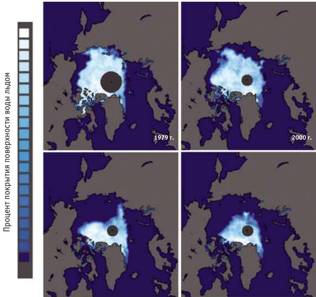
Рис. 2.8.2. Карты арктических льдов (летний минимум, наблюдающийся в сентябре).
