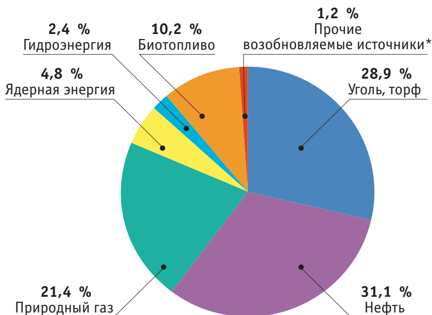
Рис. 3.1.4. Доля основных источников энергии в целом по миру, 2013 год.
