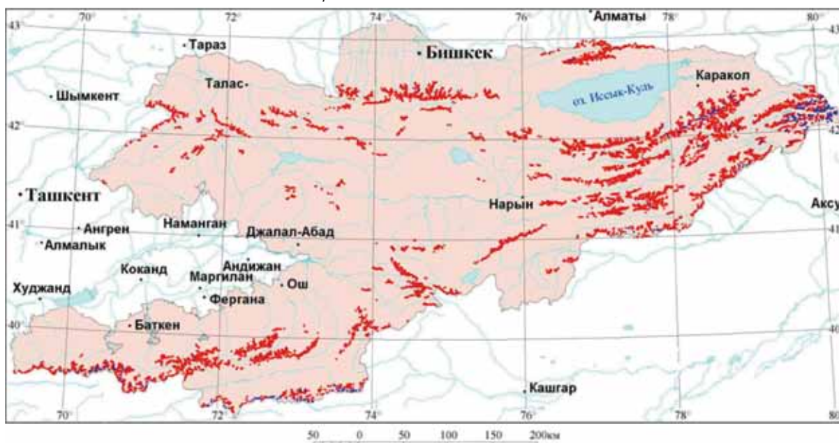
Рис. 2.4.5. Прогноз состояния оледенения в 2100 г. относительно 1960-х годов.
