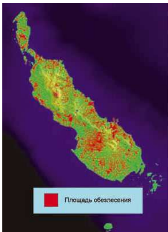
Рис. 2.3.15. Территории острова Бугенвиль (Папуа Новая Гвинея), потерявшие лесной покров за 1972–2002 годы.
