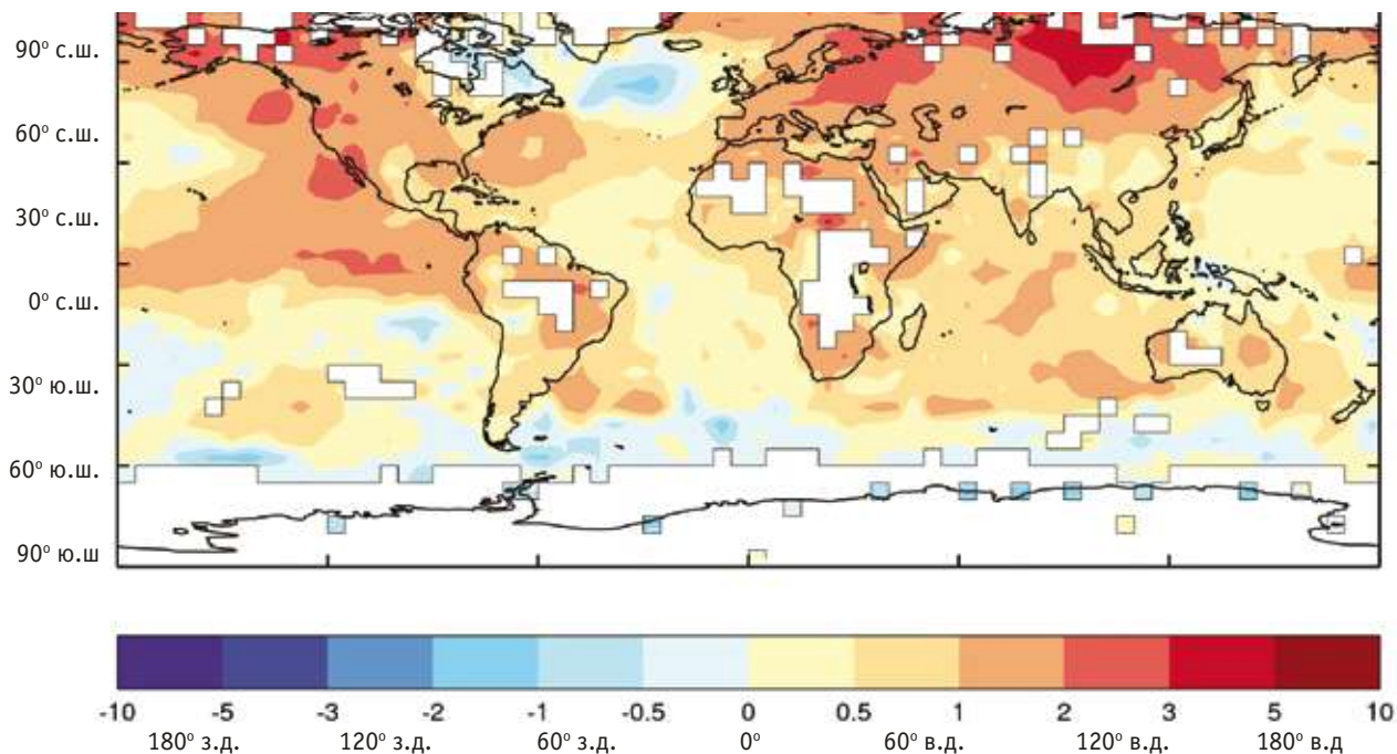
Рис. 1.4.1. Карта показывает, на сколько градусов изменилась температура в разных регионах Земли к 2015 году по сравнению со средним значением за период с 1961 по 1990 годы.
